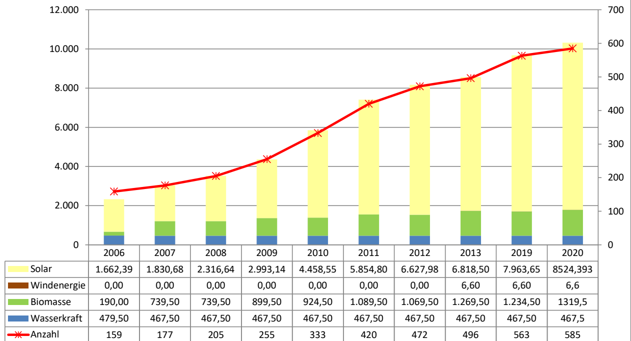
Entwicklung der EEG-Anlagenanzahl bzw. der Anschlussleistung im Netzgebiet der EVG Perlesreut e.G.
