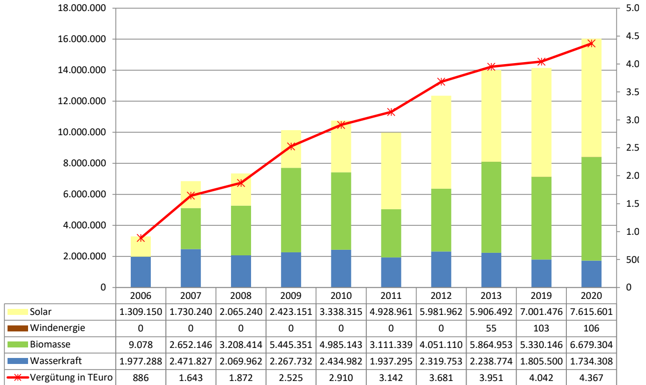
Entwicklung der EEG-Einspeisung bzw. der EEG-Vergütung im Netzgebiet der EVG Perlesreut e.G.
